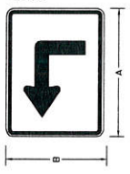
แสดงขนาดป้ายระบุทิศทาง นล-1 ถึง นล-14
